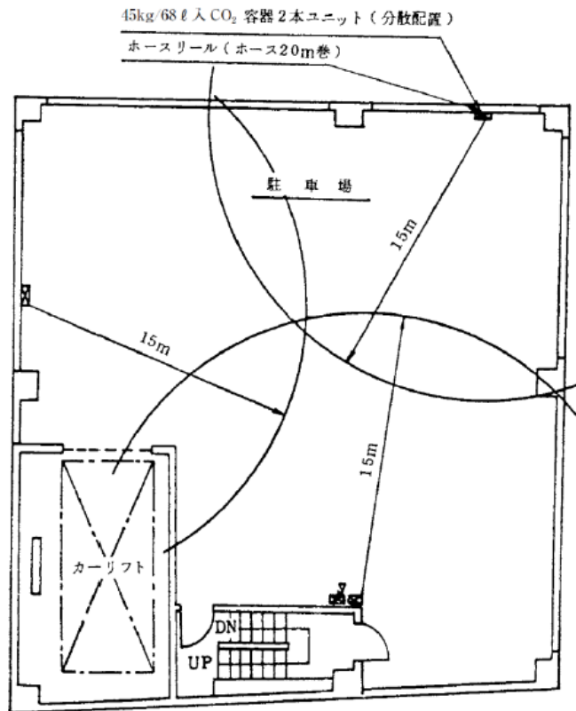
平面図
