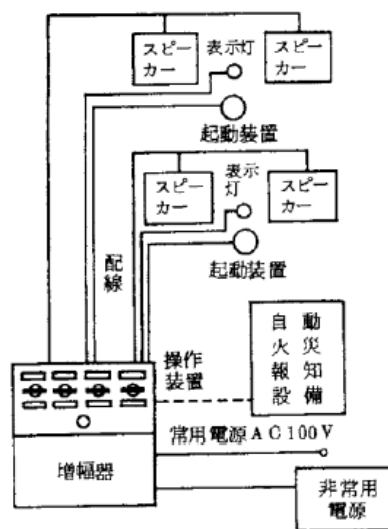
放送設備の構成図
