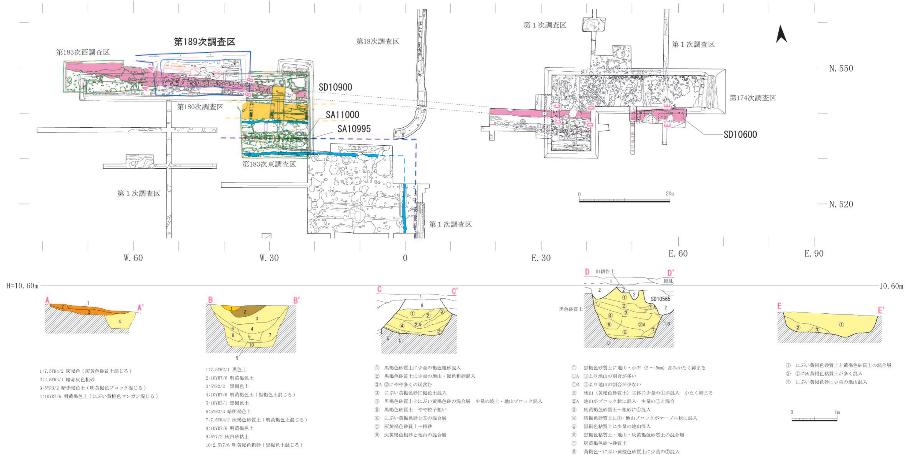
図3 古代溝平面図[1:500]・断面図[1:50]
