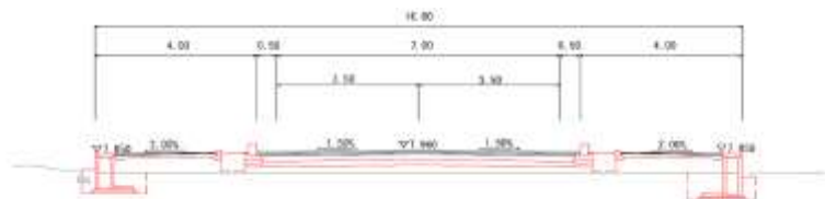
標準断面図
