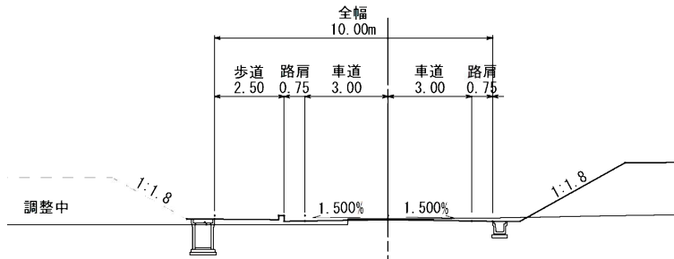
A-A断面 道路整備標準断面図
