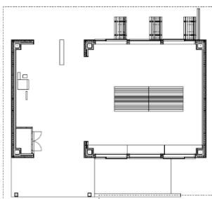
地域交流スペース平面図
