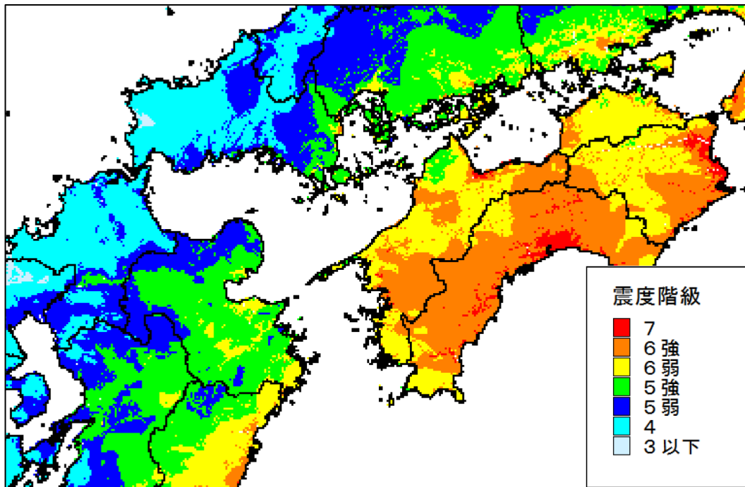
南海トラフ巨大地震の震度分布図（陸側ケース、内閣府被害想定から抜粋）
