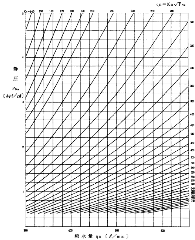
図3—11 流水表
