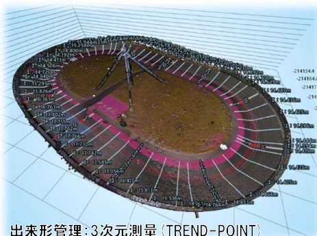
出来形管理：3次元測量（TREND-POINT）
