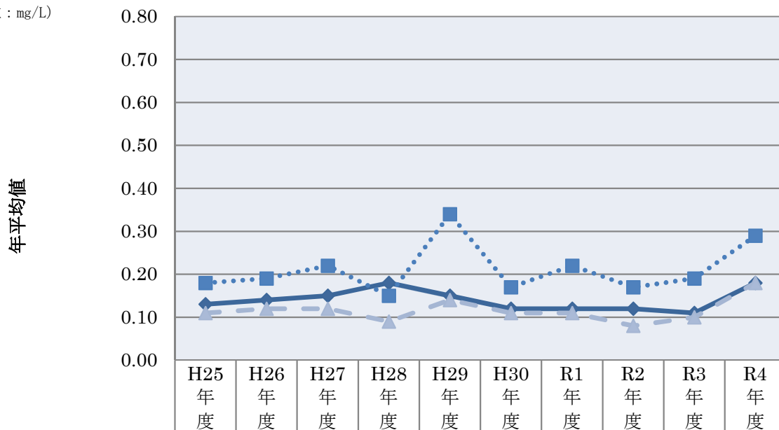
グラフ3(2)-1 全窒素の経年変化
