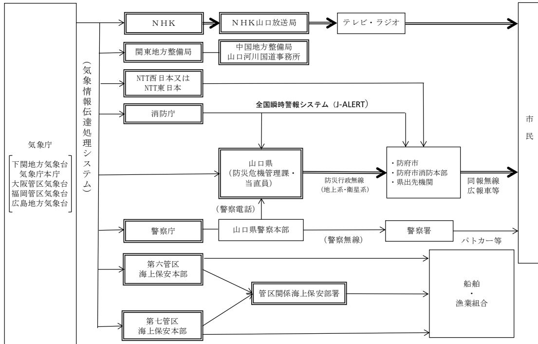
【気象台から市民までの伝達系統図】
