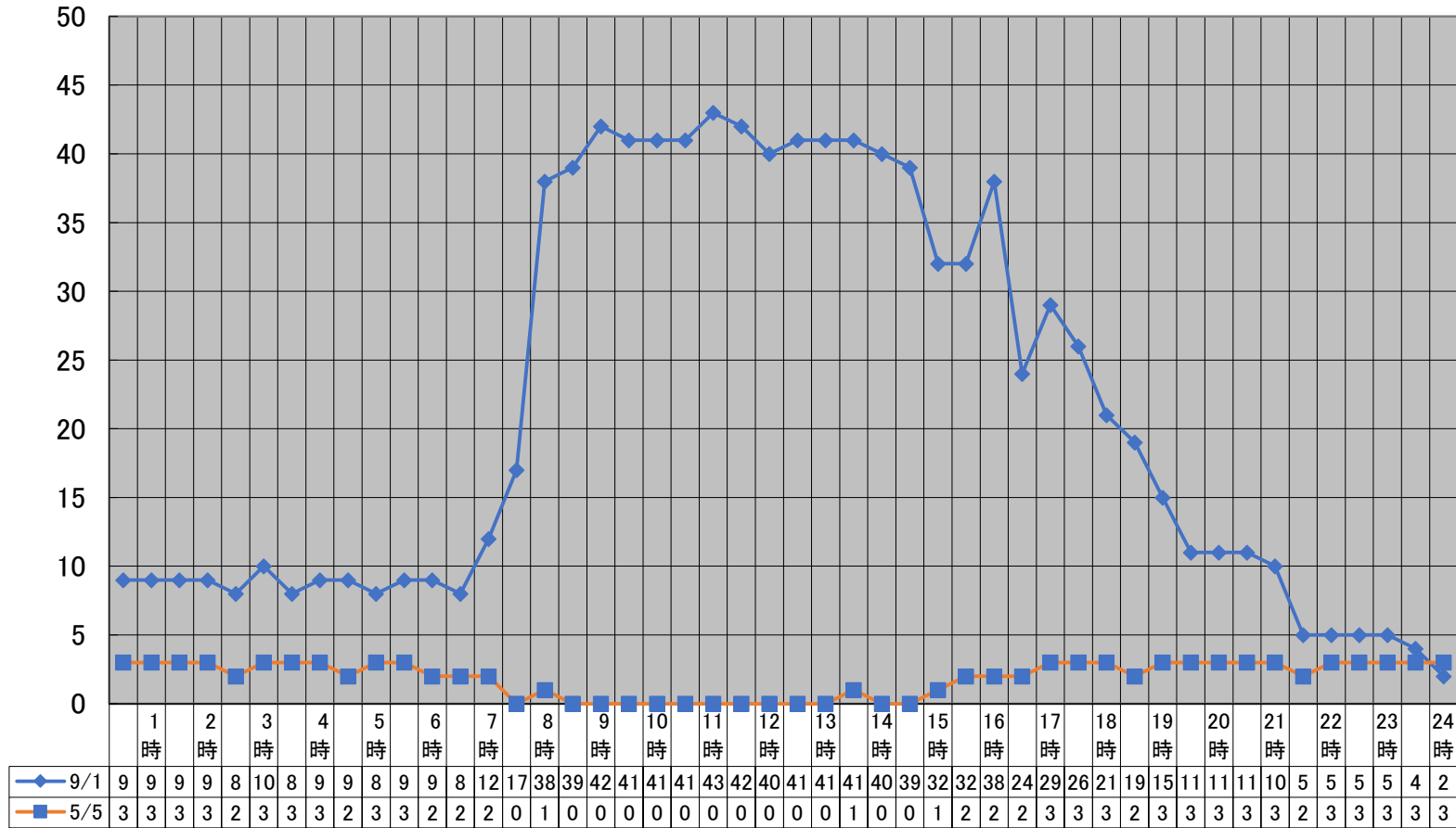
kWh 令和7年4月から令和8年3月までの最大使用電力量の日負荷曲線(最大月及び最小月) (kWh) 【右田中学校】
