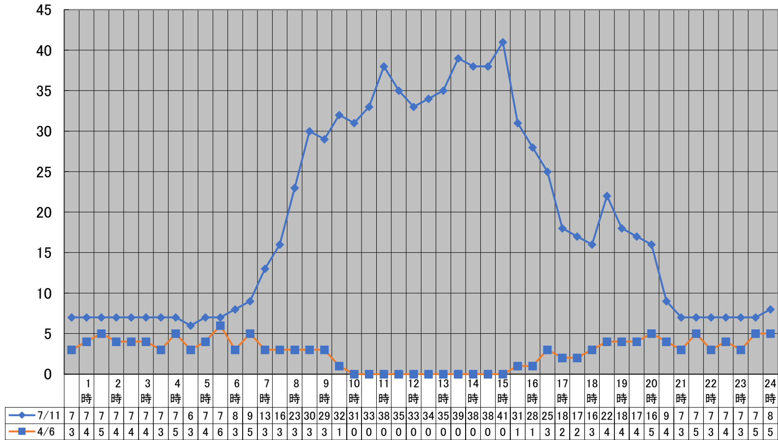
kWh 令和7年4月から令和8年3月までの最大使用電力量の日負荷曲線(最大月及び最小月) (kWh) 【大道小学校】
