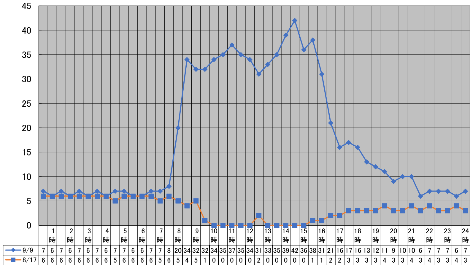
kWh 令和7年4月から令和8年3月までの最大使用電力量の日負荷曲線(最大月及び最月) (kWh) 【中関小学校】
