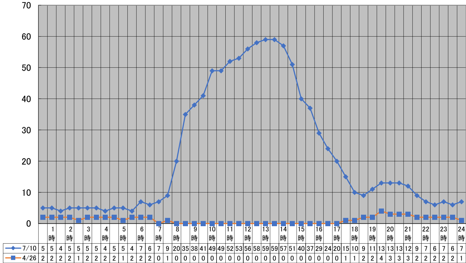
kWh 令和7年4月から令和8年3月までの最大使用電力量の日負荷曲線(最大月及び最小月) (kWh) 【佐波中学校】
