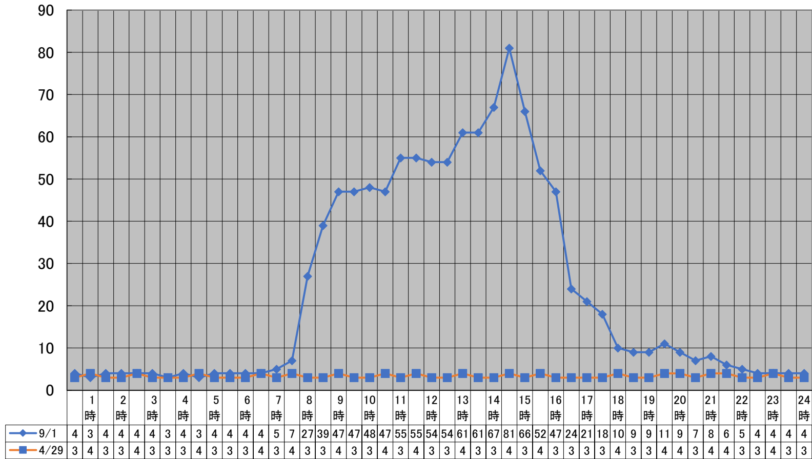
kWh 令和7年4月から令和8年3月までの最大使用電力量の日負荷曲線(最大月及び最小月) (kWh) 【小野小学校】
