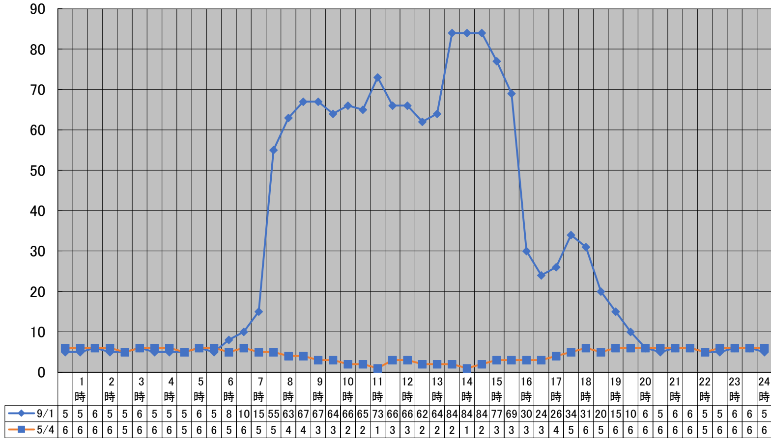
kWh 令和7年4月から令和8年3月までの最大使用電力量の日負荷曲線(最大月及び最小月) (kWh) 【勝間小学校】
