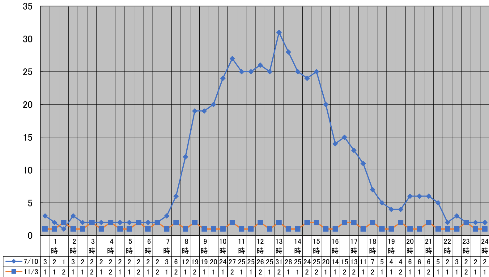
kWh 令和7年4月から令和8年3月までの最大使用電力量の日負荷曲線(最大月及び最小月) (kWh) 【小野中学校】
