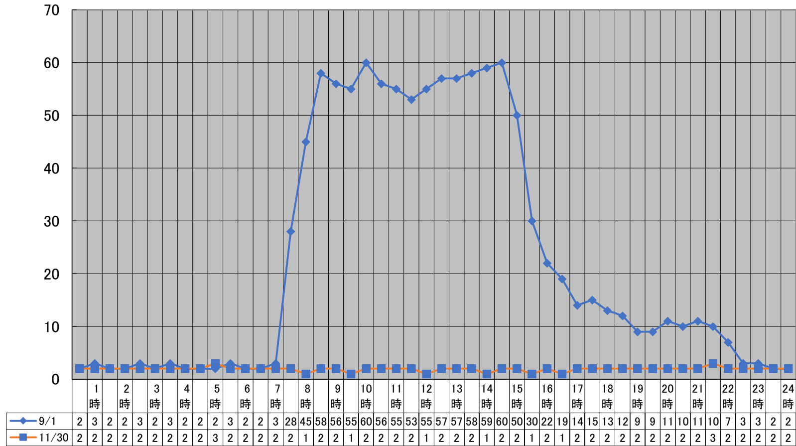
kWh 令和7年4月から令和8年3月までの最大使用電力量の日負荷曲線(最大月及び最小月) (kWh) 【牟礼南小学校】
