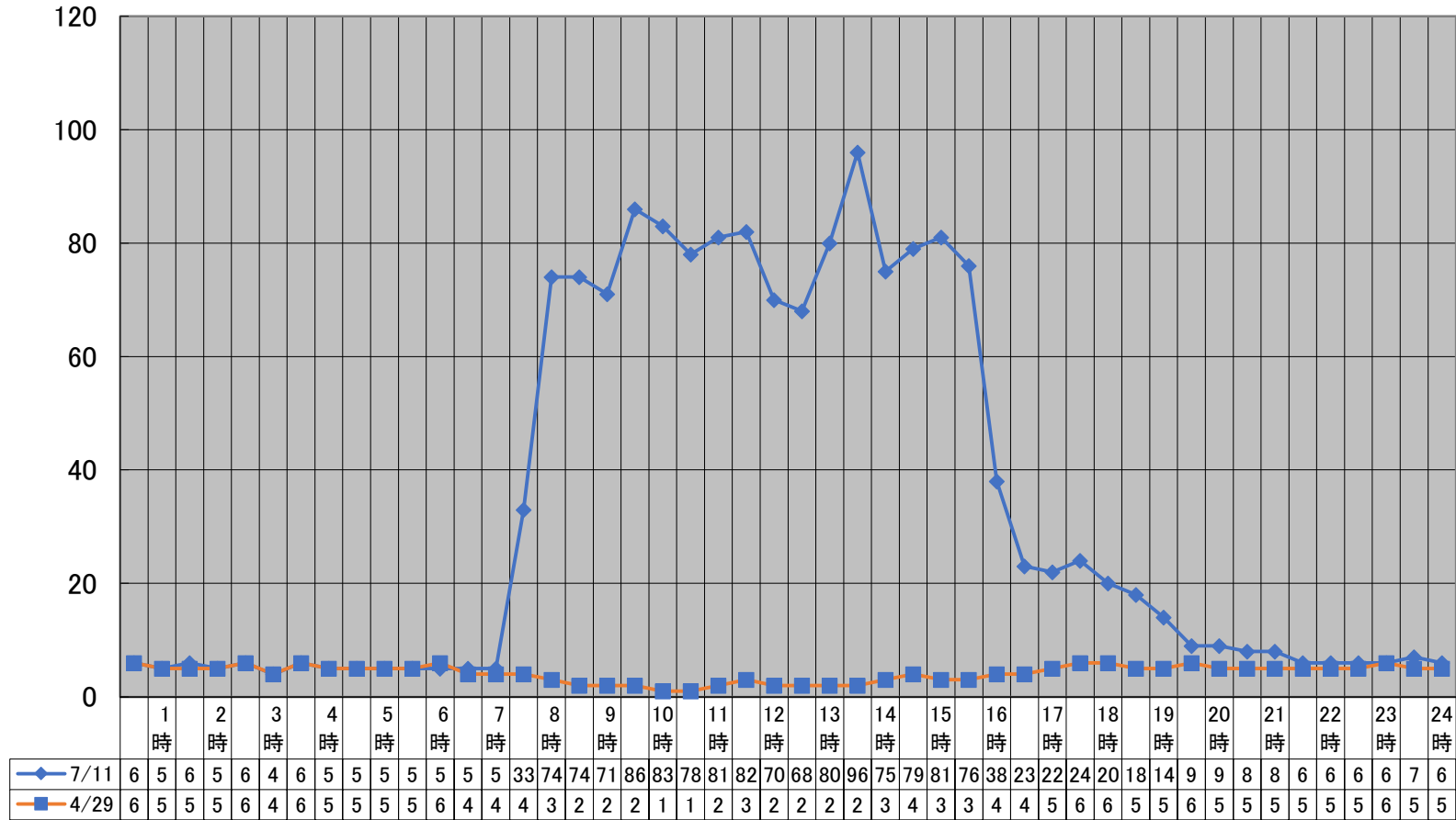
kWh 令和7年4月から令和8年3月までの最大使用電力量の日負荷曲線(最大月及び最小月) (kWh) 【右田小学校】
