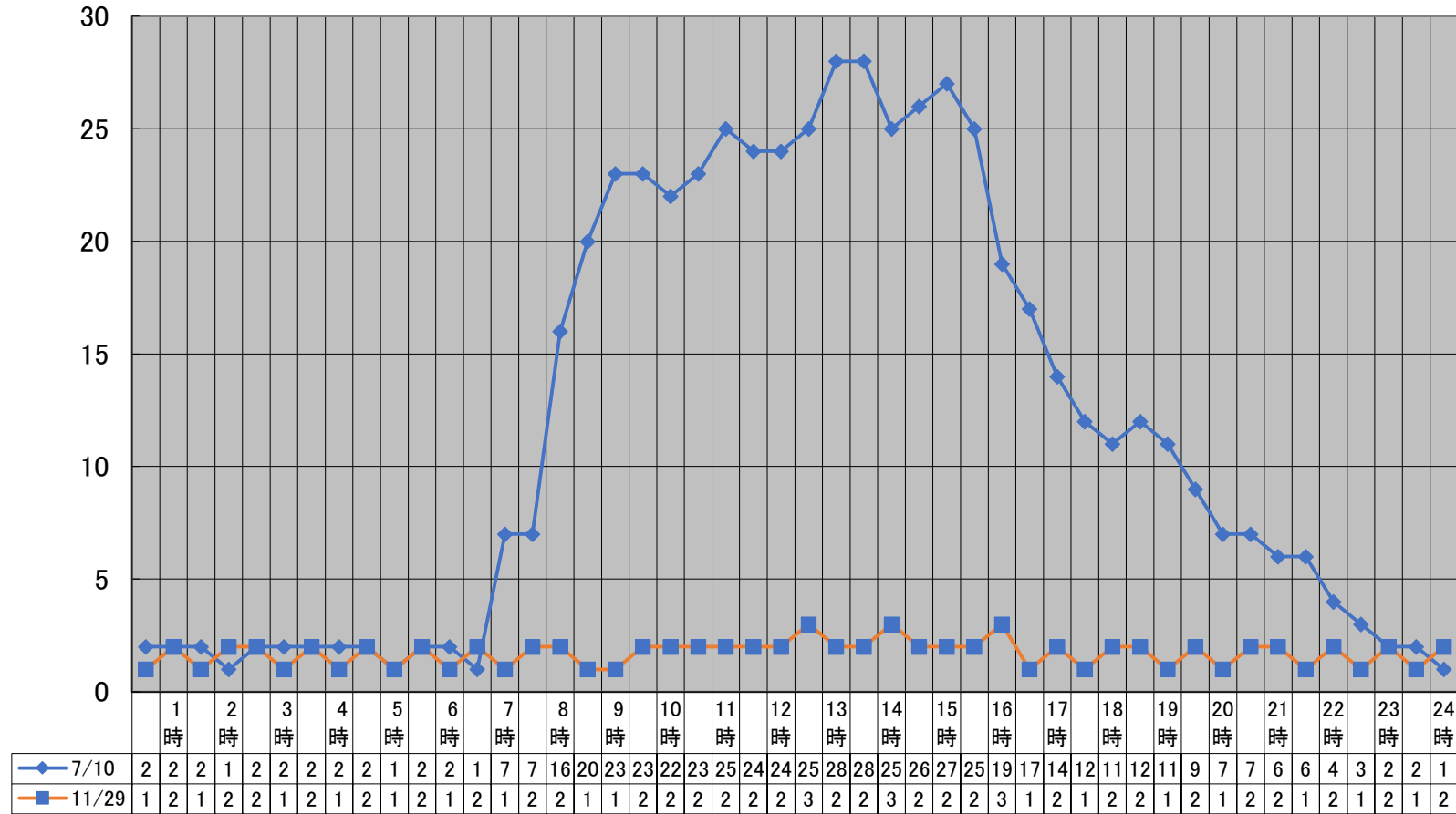
kWh 令和7年4月から令和8年3月までの最大使用電力量の日負荷曲線(最大月及び最小月) (kWh) 【牟礼中学校】
