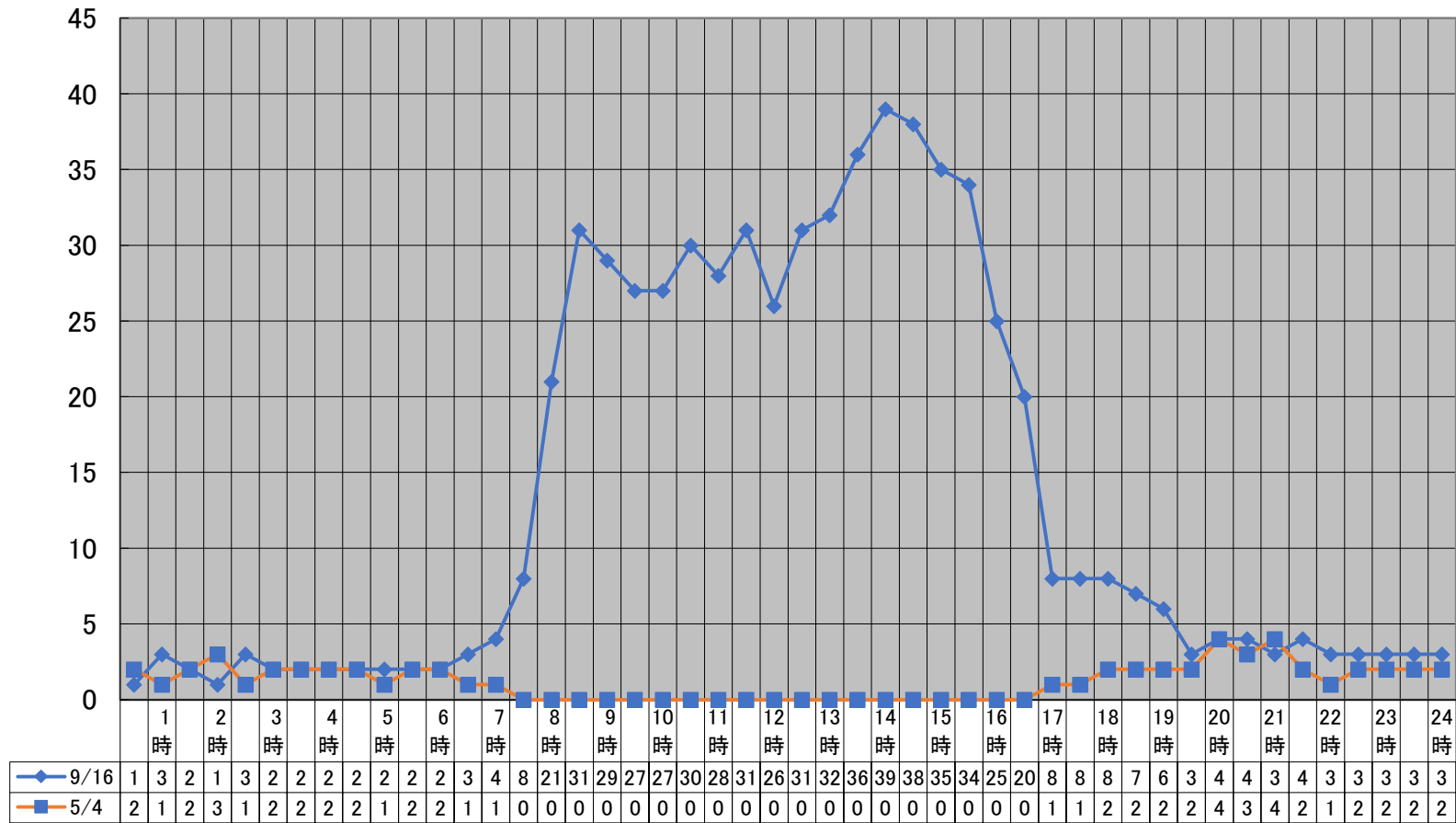
kWh 令和7年4月から令和8年3月までの最大使用電力量の日負荷曲線(最大月及び最小月) (kWh) 【西浦小学校】
