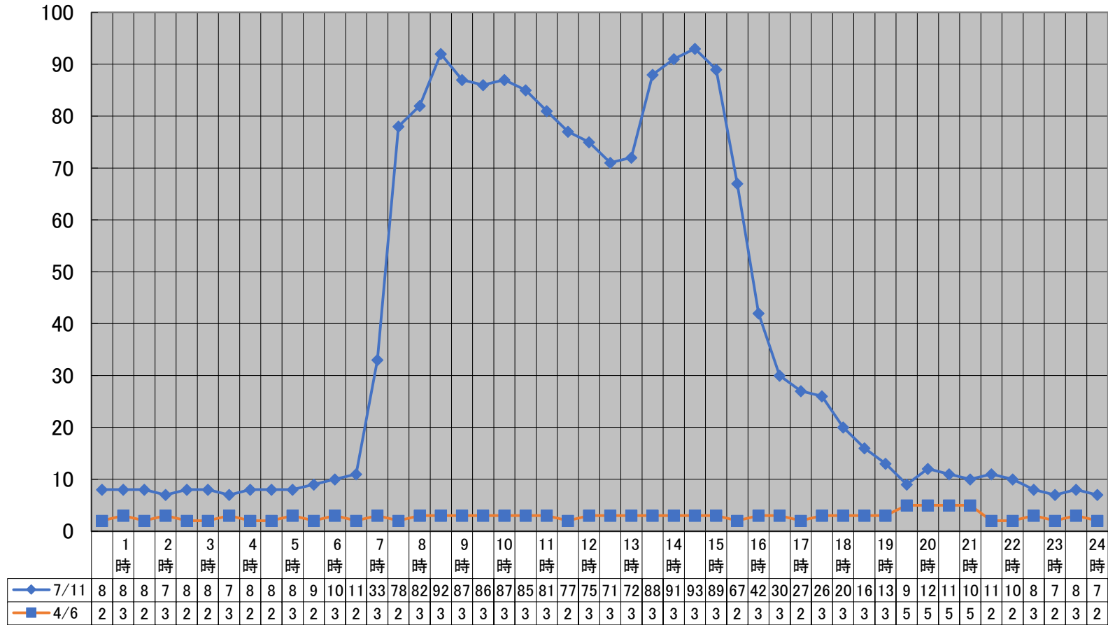
kWh 令和7年4月から令和8年3月までの最大使用電力量の日負荷曲線(最大月及び最小月) (kWh) 【華浦小学校】
