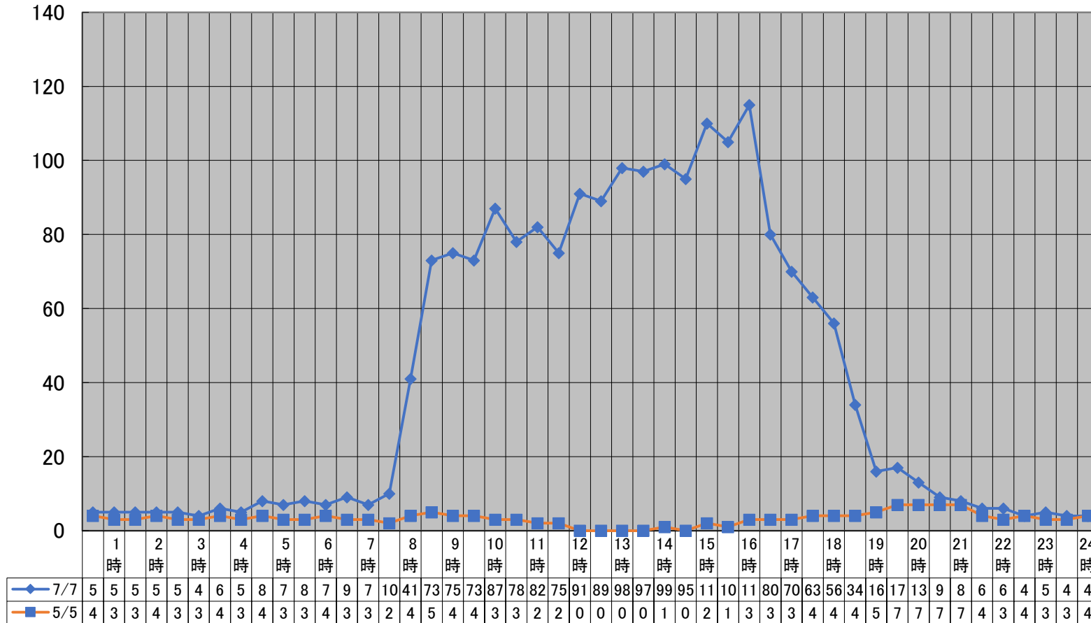
kWh 令和7年4月から令和8年3月までの最大使用電力量の日負荷曲線(最大月及び最小月) (kWh) 【桑山中学校】
