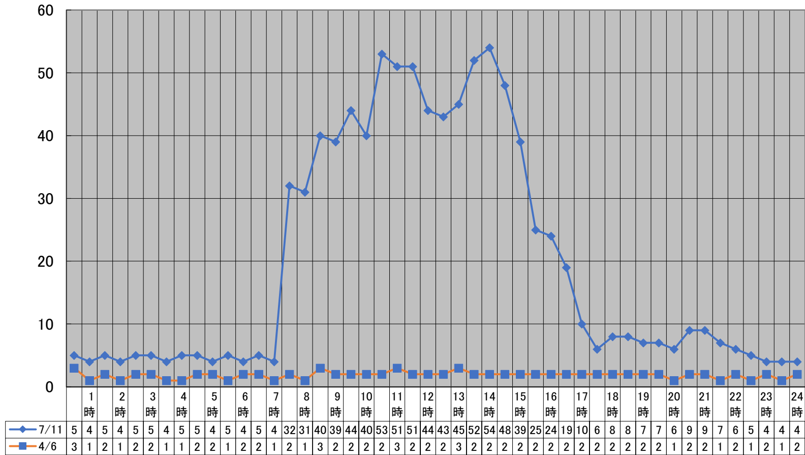
kWh 令和7年4月から令和8年3月までの最大使用電力量の日負荷曲線(最大月及び最小月) (kWh) 【玉祖小学校】
