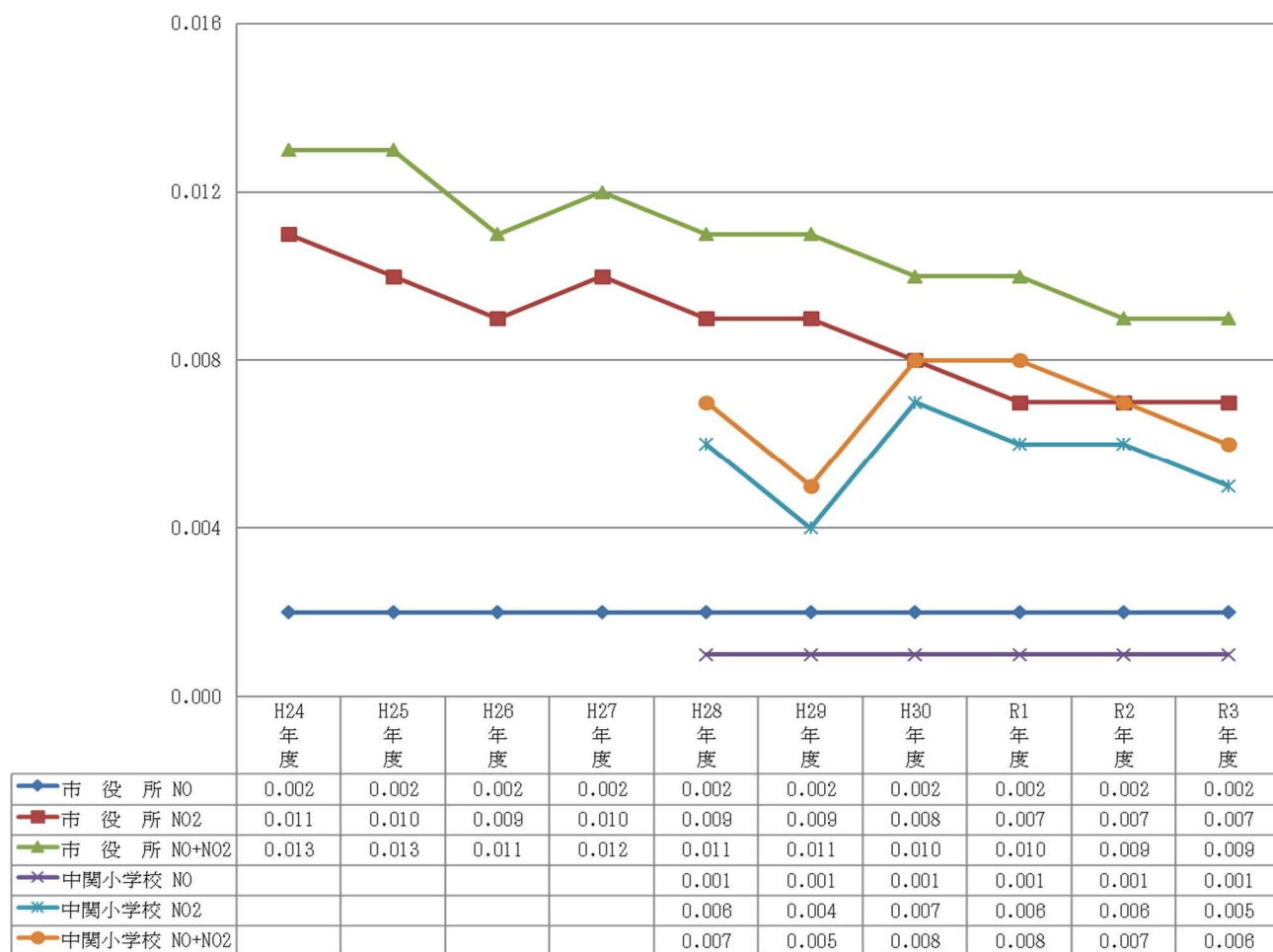
グラフ3(2)オ 窒素酸化物 (NO, NO 2 , NO+NO 2 ) 濃度年平均値の経年変化
