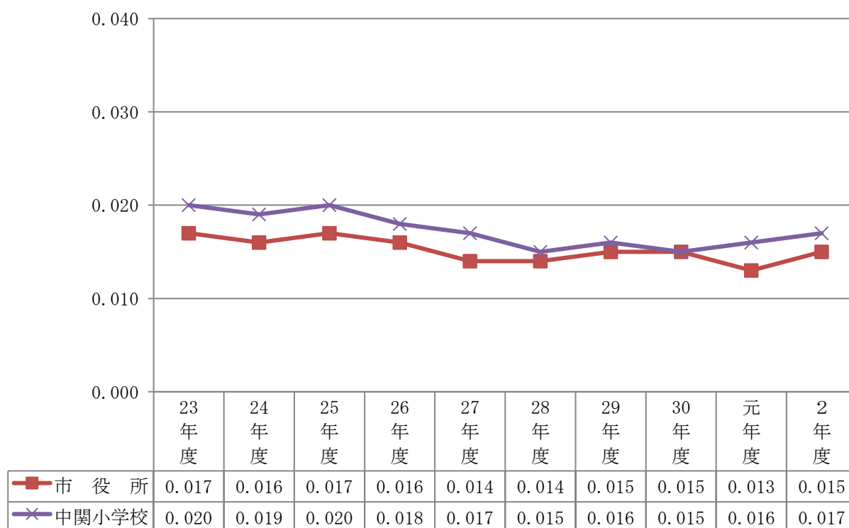
グラフ3(2)イ 浮遊粒子状物質濃度年平均値の経年変化
