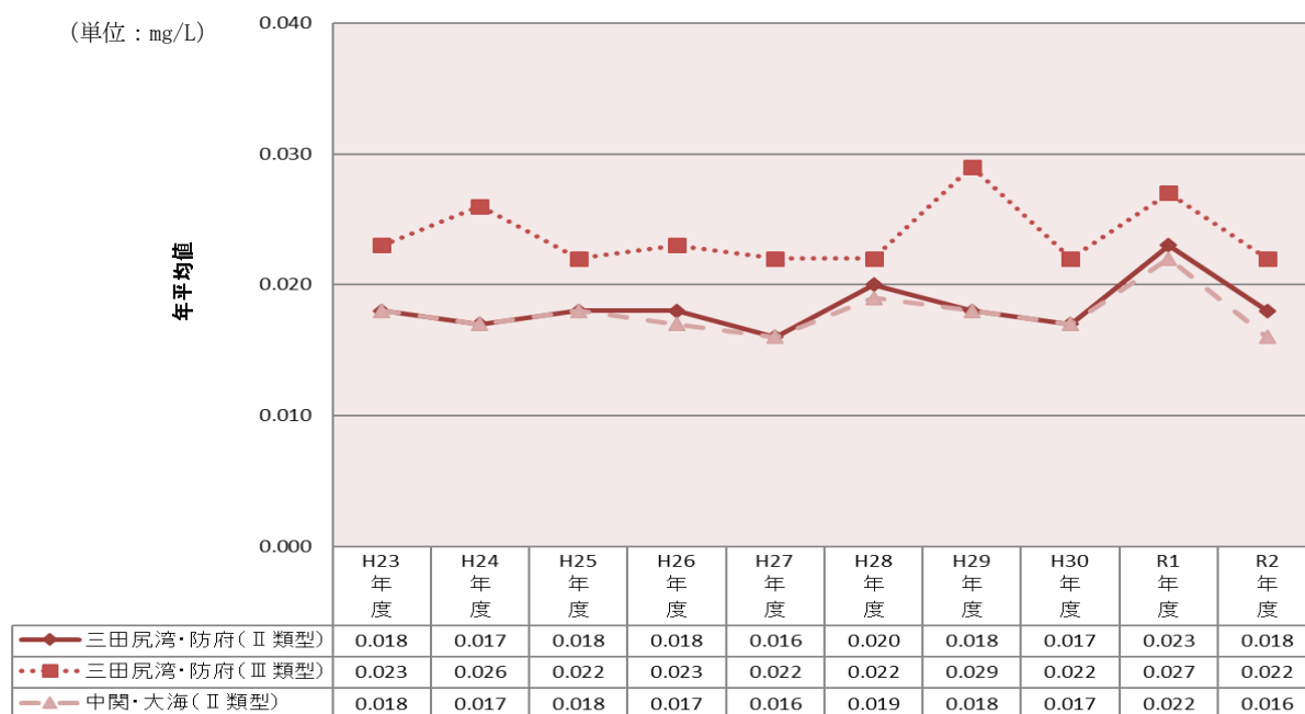
グラフ3(2)-2 全磷の経年変化
