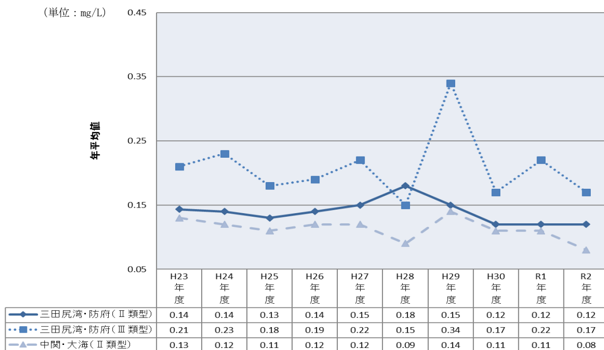
グラフ3(2)-1 全窒素の経年変化
