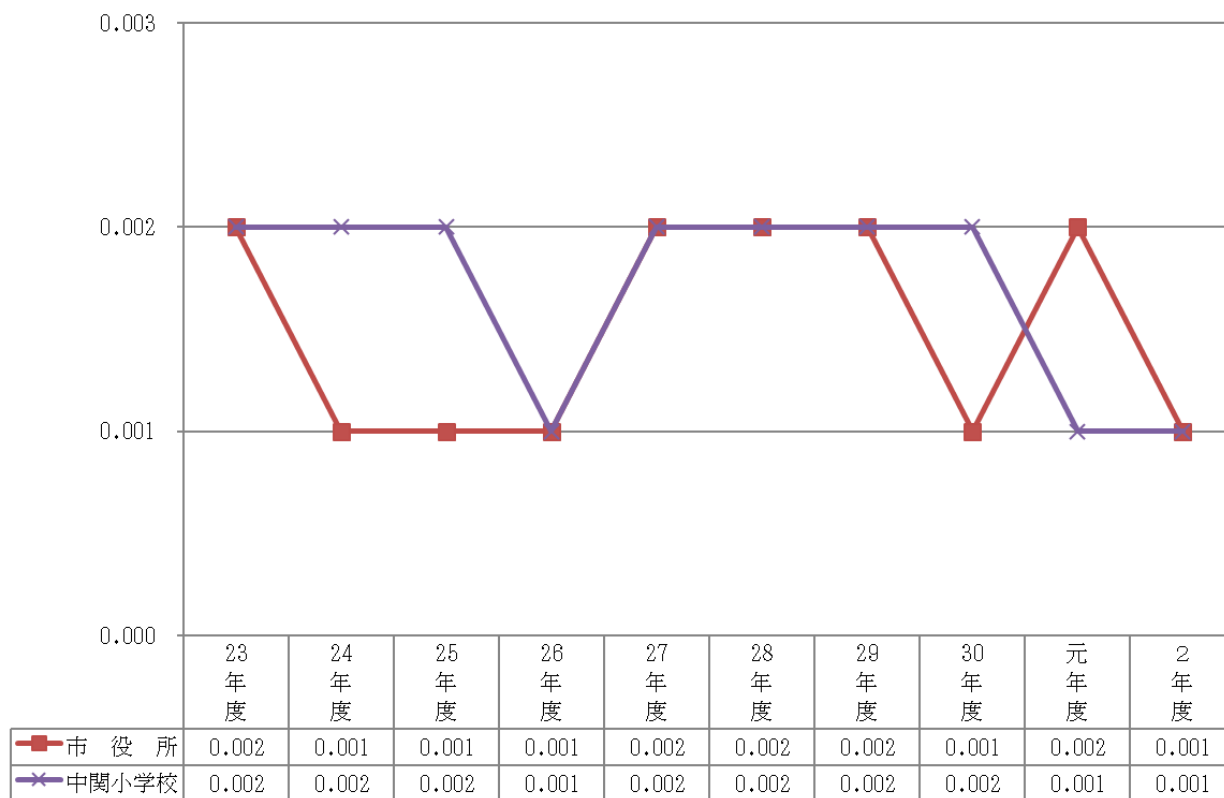
グラフ 3 (2) ア 二酸化硫黄濃度年平均値の経年変化
