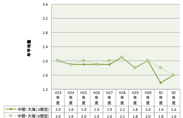
中関・大海海域におけるCODの経年変化(単位: mg/L)
