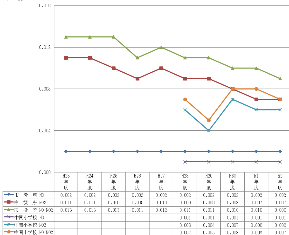
グラフ3(2)オ 窒素酸化物 (NO, NO 2 , NO+NO 2 ) 濃度年平均値の経年変化
